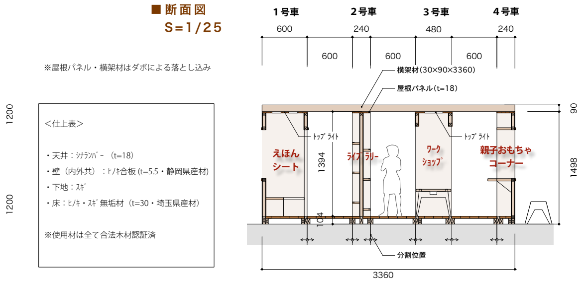
組み立て： 壁面の連結時は、 ベルクロ にて取り付く仕上パネルを脱着します。ボルトはM6。
